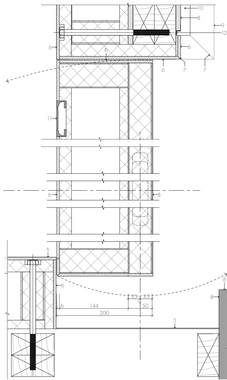
DETAIL PLAN - pivot door
